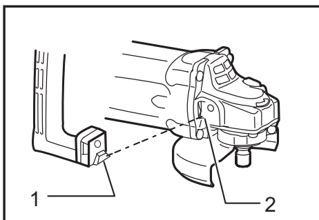
► 1. Saillie de la poignée arceau 2. Orifice de couplage dans le carter d'engrenage
