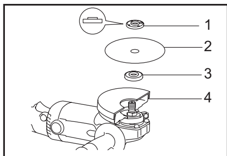
► 1. Contre-écrou 2. Meule à découper 3. Bague interne 4. Carter de meule à découper
